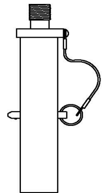
UPPER MAST ADAPTER P/N: RAMI48-10 QTY.: 1
